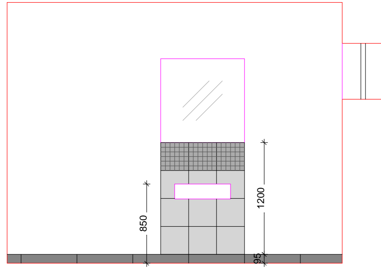
POHLED DD:
