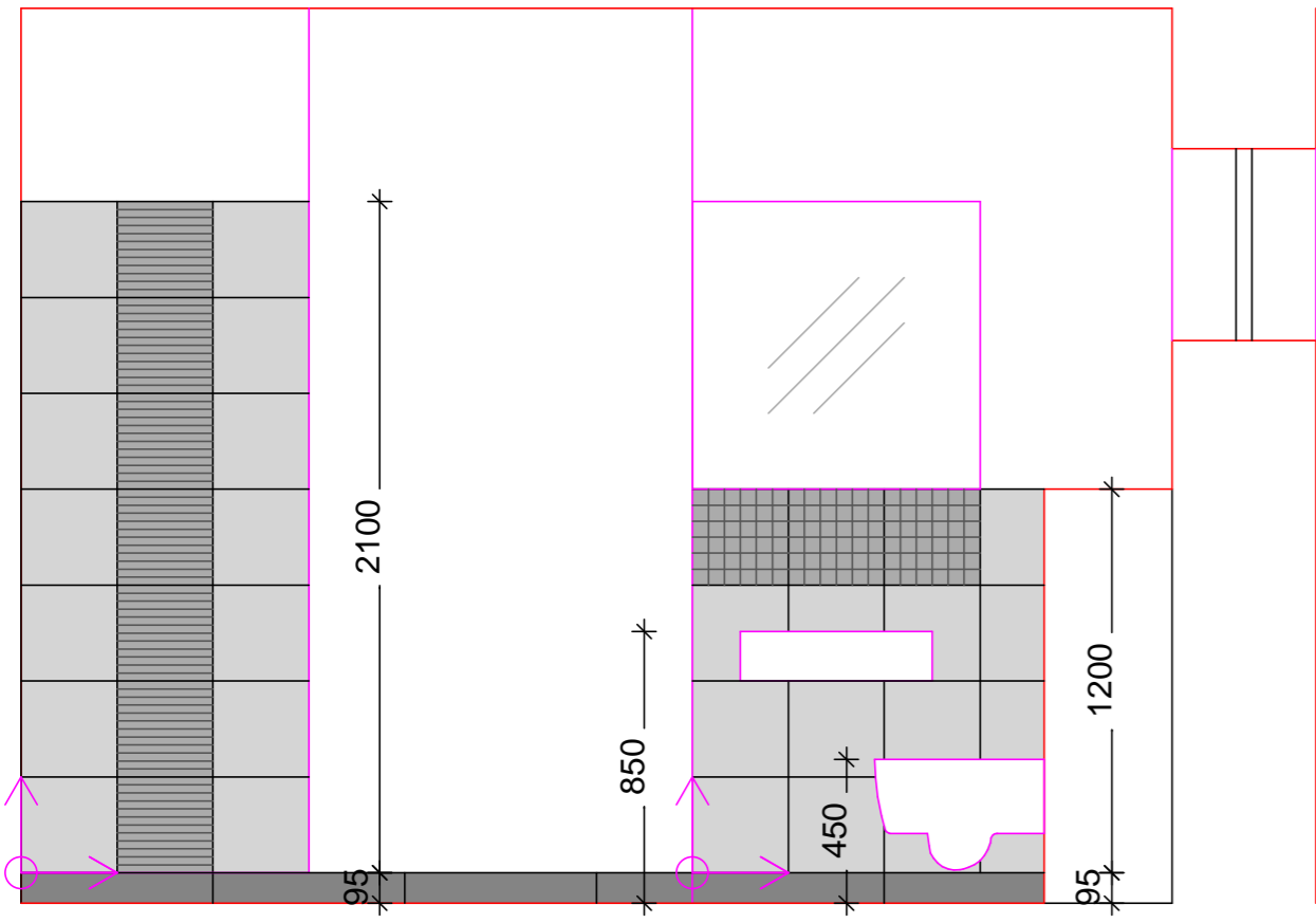
POHLED AA:
