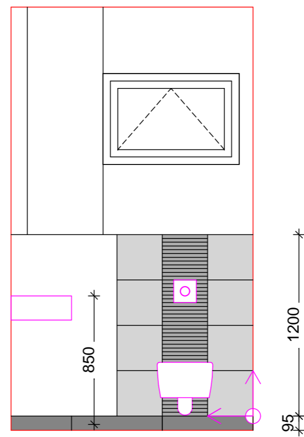
POHLED BB:
