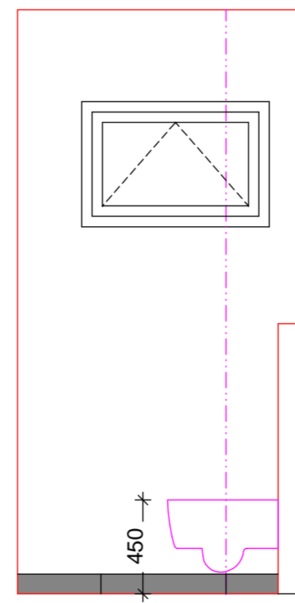
POHLED CC:
