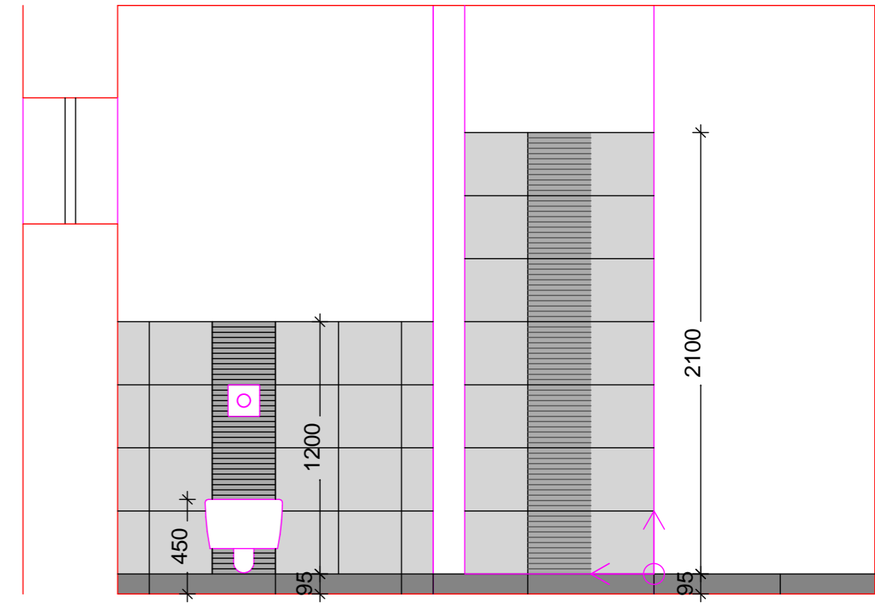
POHLED EE:
