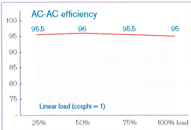
Graf 1 - Účinnost UPS
