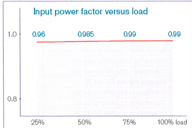
Graf 2 – Průběh vstupního PF
