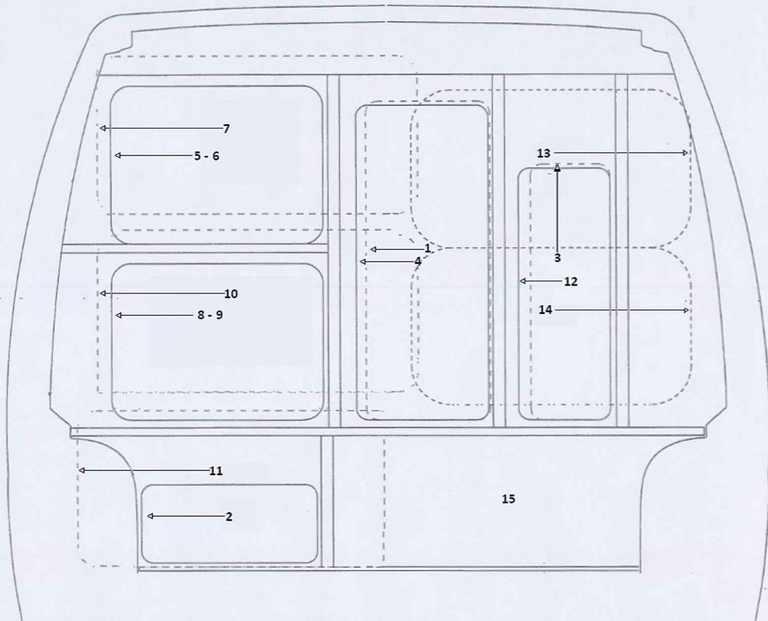
Pohled na zadní část vozidla v řezu
