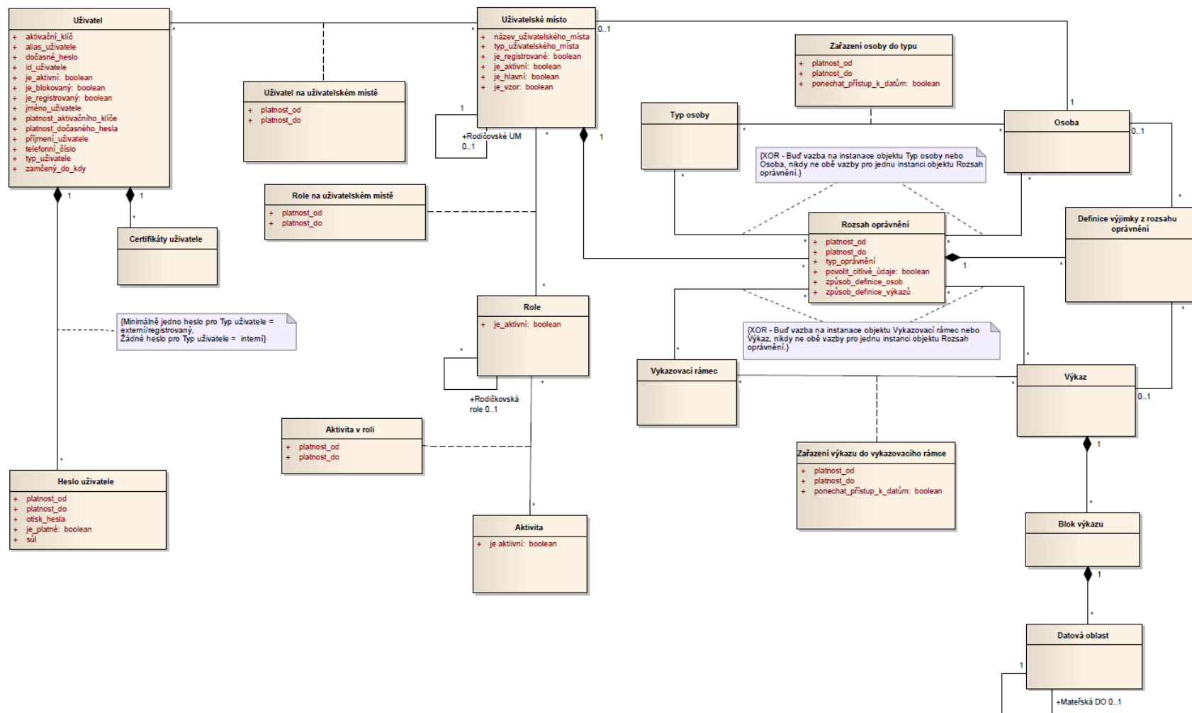
Obrázek 1 - Objektový model pro oblast Uživatelé a Oprávnění
