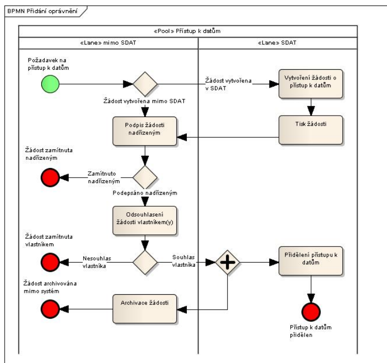
Obrázek 2 - Proces přidělení oprávnění přístupu k datům
