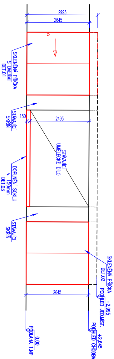
POHLED NA STĚNU Z CHODBY M 1:100
