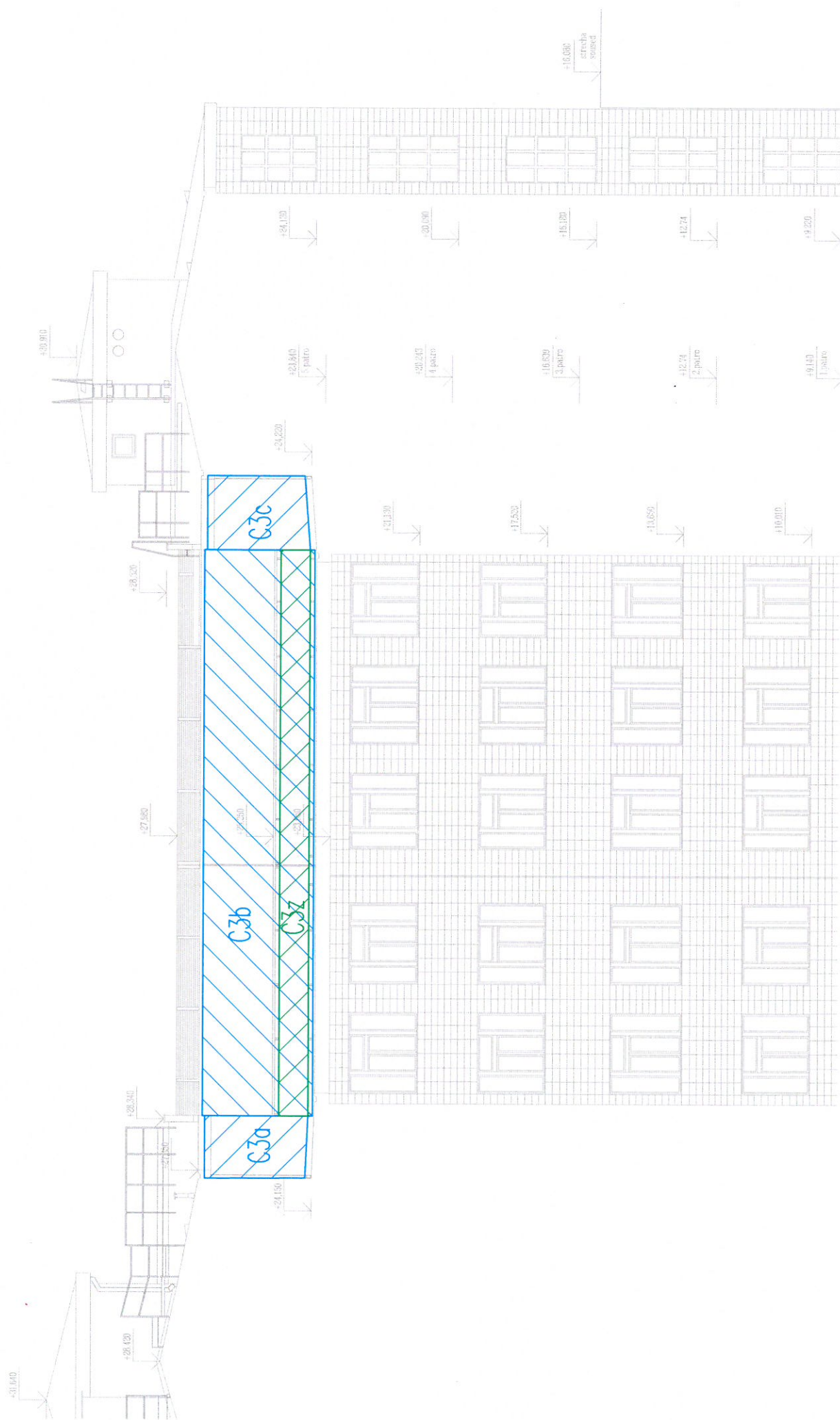
Renovace omítkových fasád v úrovni 5P pohled na fasádu č. 29 - M1:10
