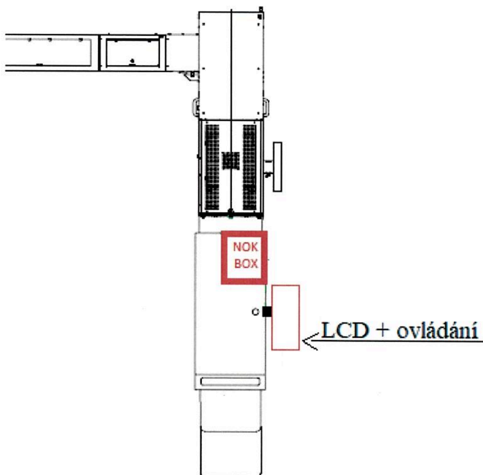
Obrázek 1 Umístění NOK boxu a ovládacích prvků zařízení optické kontroly bankovek do místa plnění ČNB Praha
