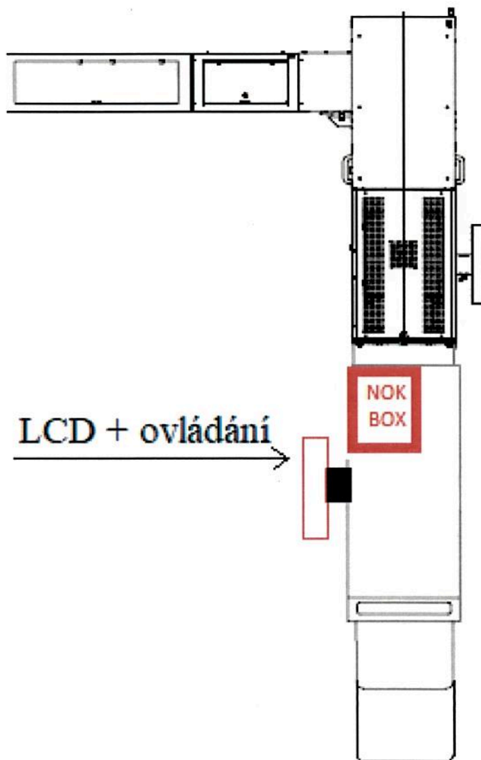
Obrázek 2 Umístění NOK boxu a ovládacích prvků zařízení optické kontroly bankovek do místa plnění ČNB Brno
